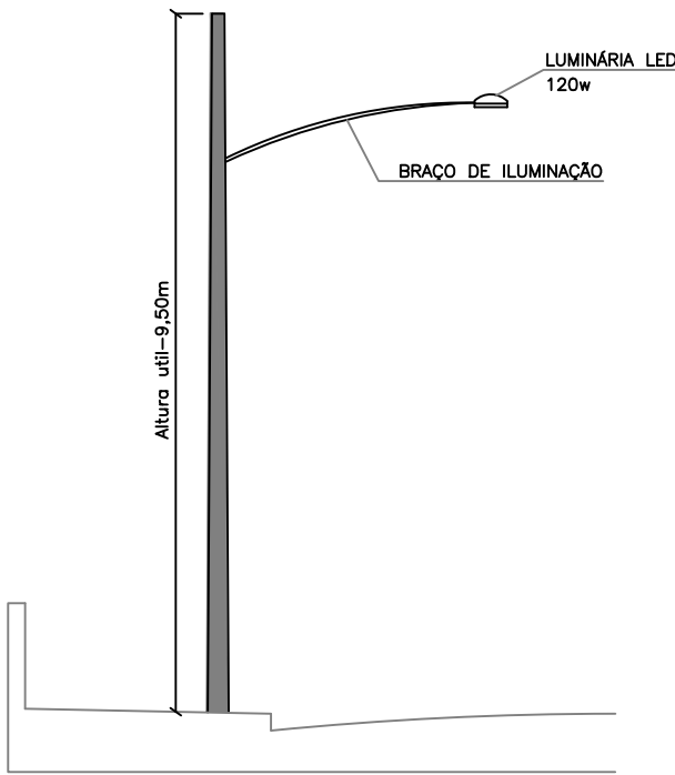
DETALHE POSTE DE LUZ NO PASSEIO s/escala
